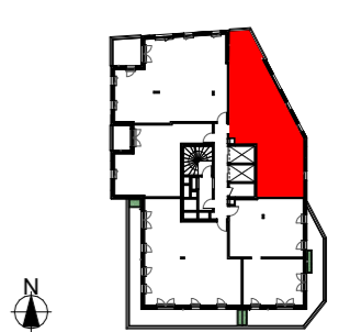
Plan étage
